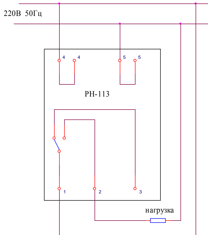
Примечание. Контакты реле показаны при обесточенном реле. Рисунок 2 – Схема подключения реле
